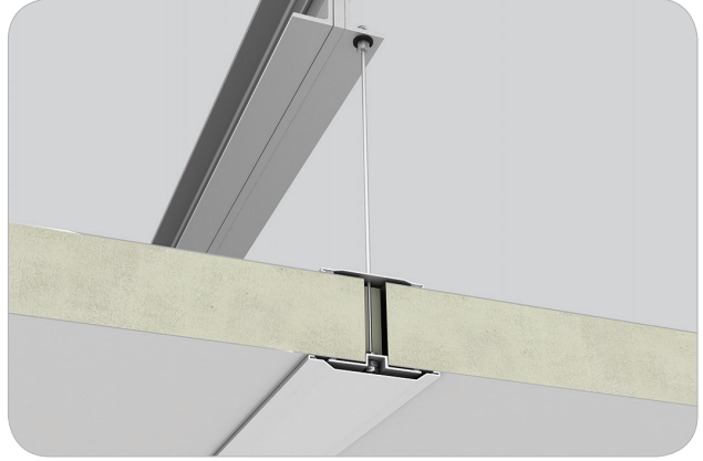
Soğuk Oda İç Köşe Tavan Detayı-2 / Cold Room Inner Corner Ceiling Detail-2
